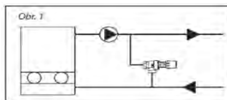
Příklad 1: Regulace přepuštěním přes topný okruh
