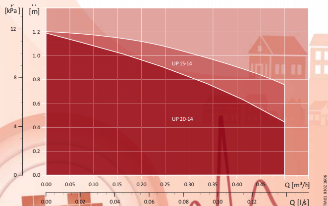
Výkonové křivky.
