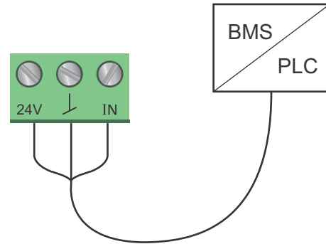
Obr. 51 Příklady externího signálu pro ovládání pomocí BMS nebo PLC
