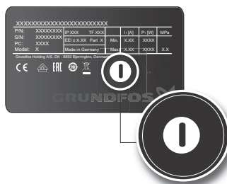
Obr. 64 Identifikace řídicího čerpadla ve zdvojeném čerpadle
