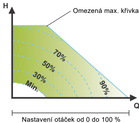
Obr. 37 Omezení výkonu a tlaku ovlivňující maximální křivku
