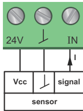
Obr. 49 Analogový vstup pro externí snímač, 4-20 mA
