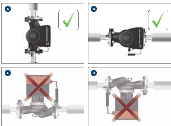
Obr. 4 Čerpadlo instalované s horizontálním hřídelem motoru
