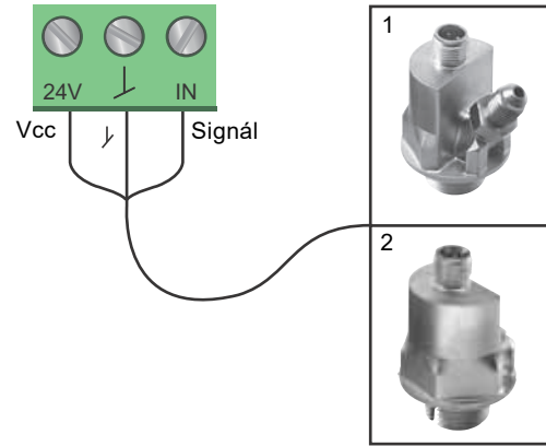
Obr. 50 Příklady externích snímačů
