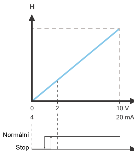
Obr. 55 "Lineární se stop", 0-10 V
