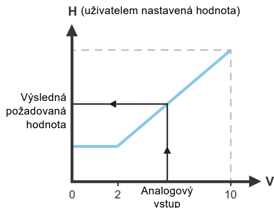
Obr. 53 "Lineární s Min.", 0-10 V
