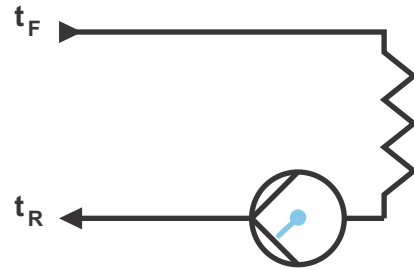
Obr. 32 Čerpadlo s interním snímačem
