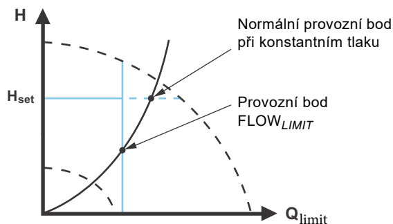
Obr. 40 Řízení na konstantní tlak pomocí funkce FLOW_{LIMIT}
