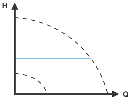
Obr. 29 Řízení na konstantní tlak
