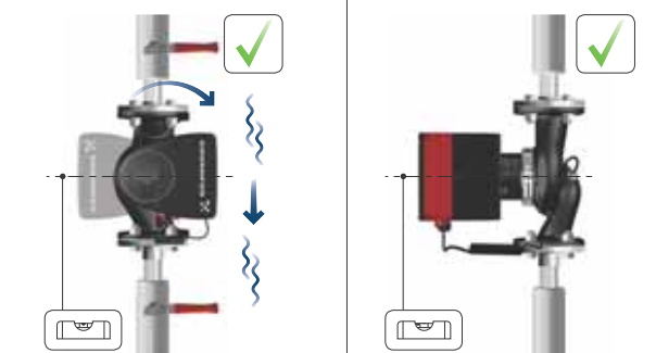
Obr. 5 Čerpadlo s řídicí jednotkou v horizontální poloze
