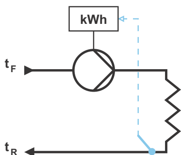
Obr. 52 MAGNA3 s vestavěným monitorem tepelné energie
