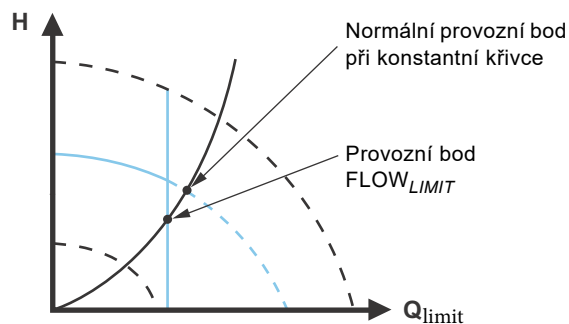
Obr. 41 Konstantní křivka pomocí funkce FLOW_{LIMIT}
