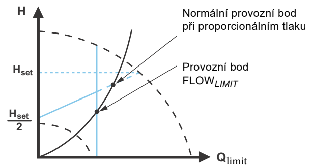
Obr. 39 Řízení na proporcionální tlak pomocí funkce FLOW_{LIMIT}
