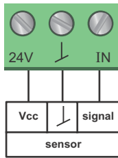
Obr. 48 Analogový vstup pro externí snímač, 0-10 V
