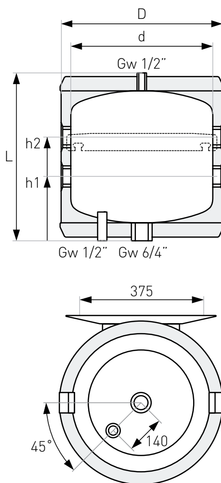
Schéma akumulční nádrže THPS 60-120IZ
